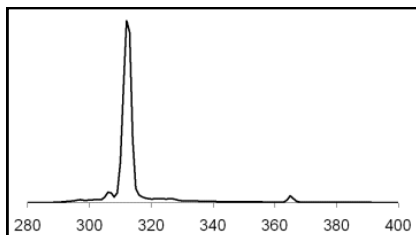
UVB-311-Spectrum
